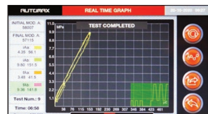
Determinación del Módulo Elástico y coeficiente de Poisson
